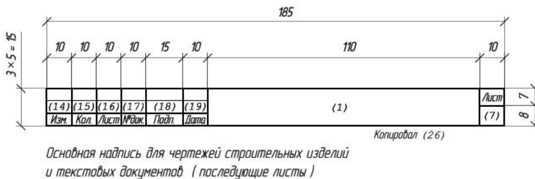
Рисунок 2. Основная надпись размером 185 x 15 на листах пояснительной записки
